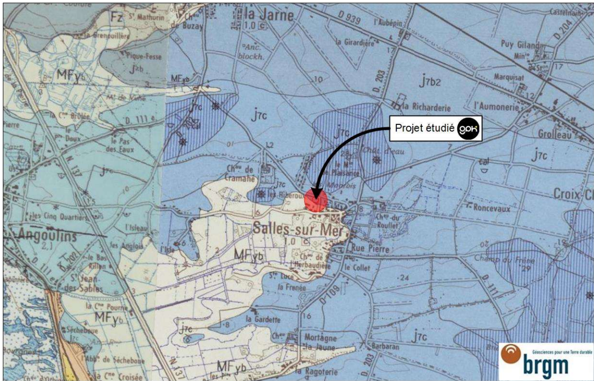
Extrait de la carte géologique (SURGÈRES) au 1/50000
